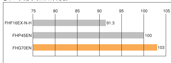
● ランプ効率 (lm/W) 比較
