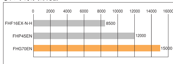
● ランプ寿命 (h) 比較
