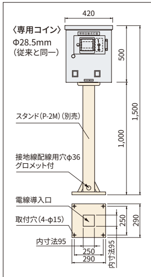
● 外形図(単位:mm) 従来品と同一寸法
