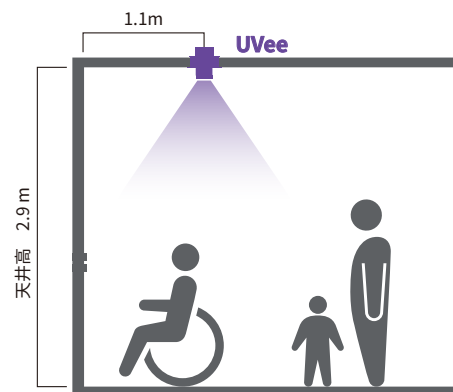
■概略断面図 北エレベーターホール
